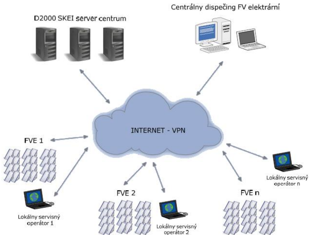
Principiálne schématické zobrazenie systému PV MONITOR
